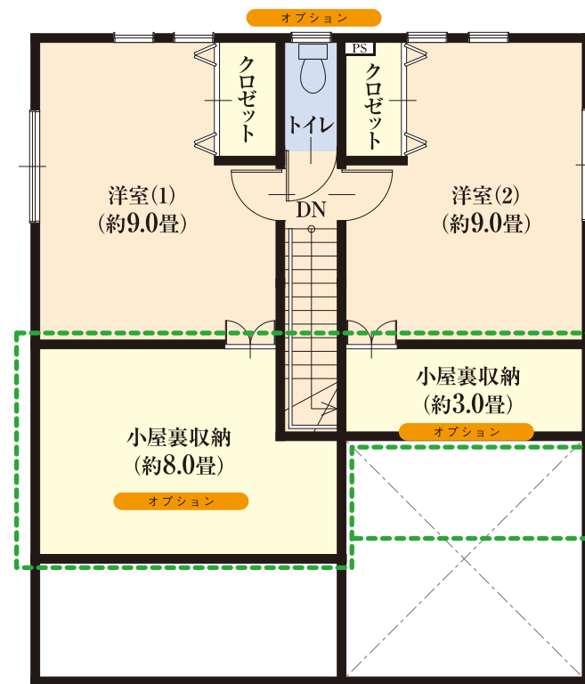
■小屋裏居室平面図
